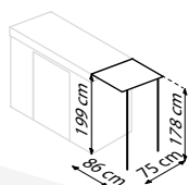
SCHLEPPDACH
